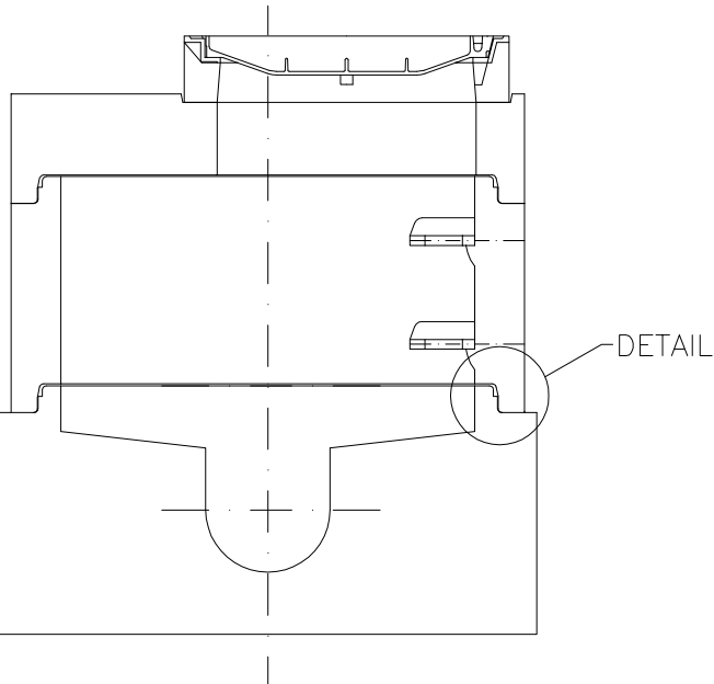
SESTAVA ŠACHTY - PŘÍKLAD
