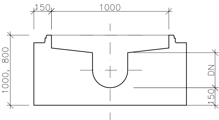
ŠACHTOVÉ DNO
