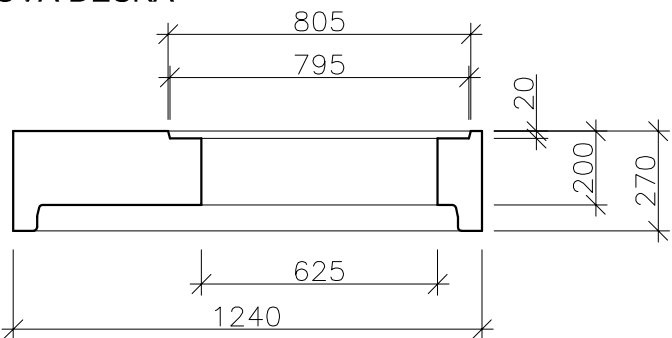
PŘECHODOVÁ DESKA
