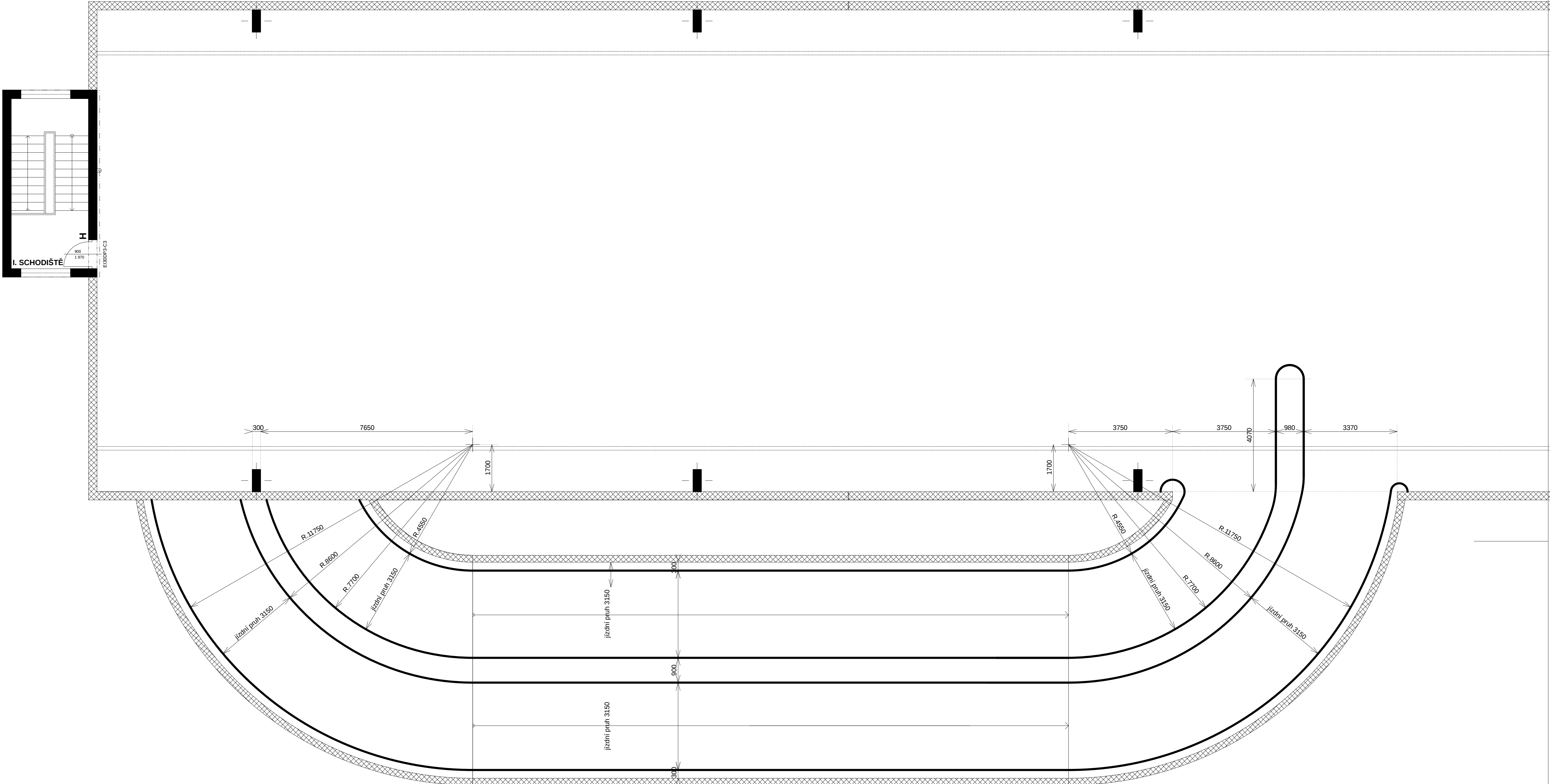
půdorysné schema 4.NP - střecha m. 1 : 75
