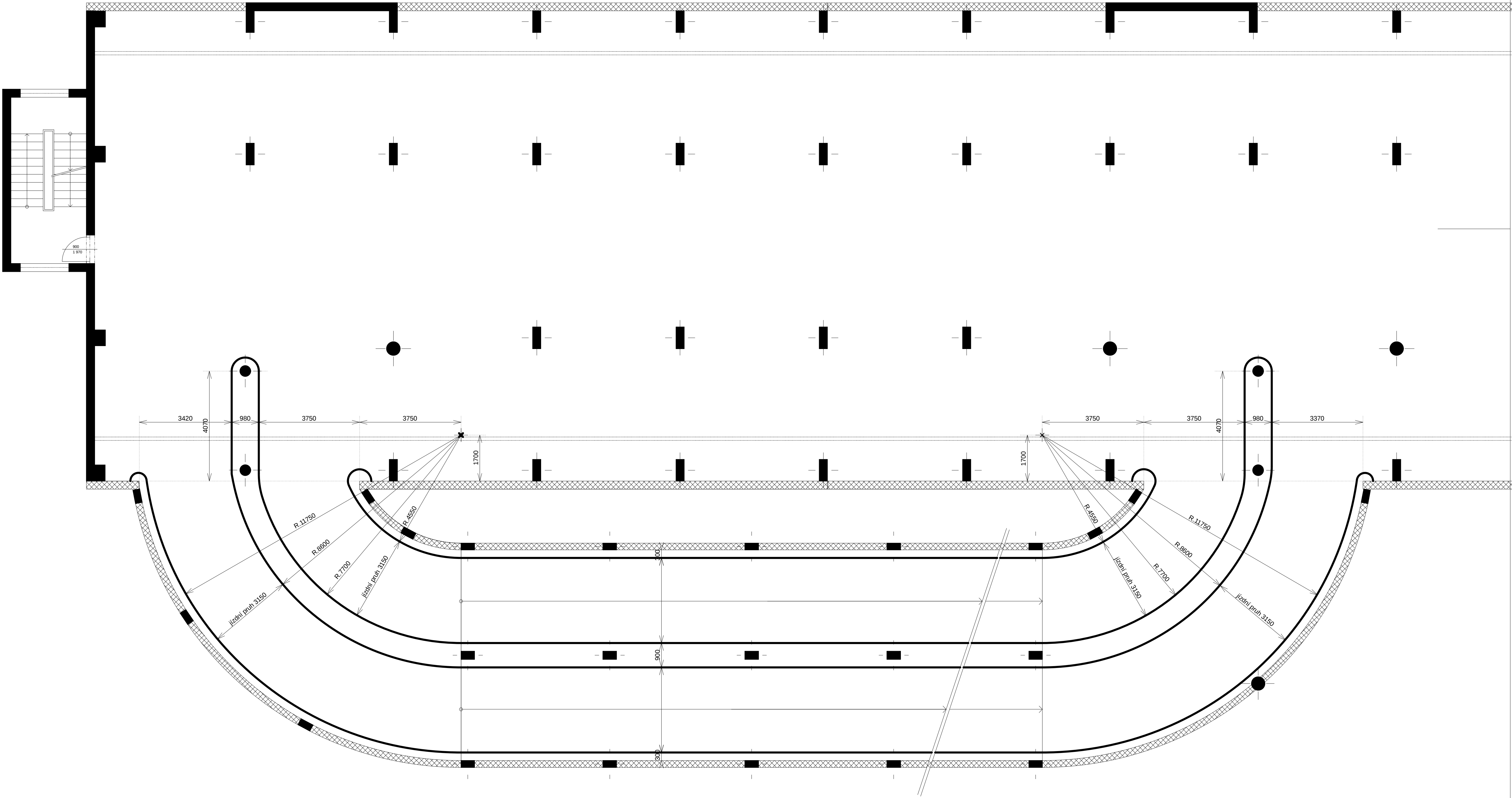
půdorysné schema 2.NP a 3.NP m. 1 : 75
