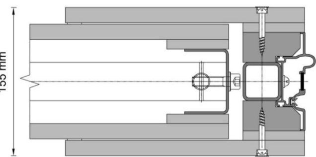
Ukončení teleskopického panelů u stěny
