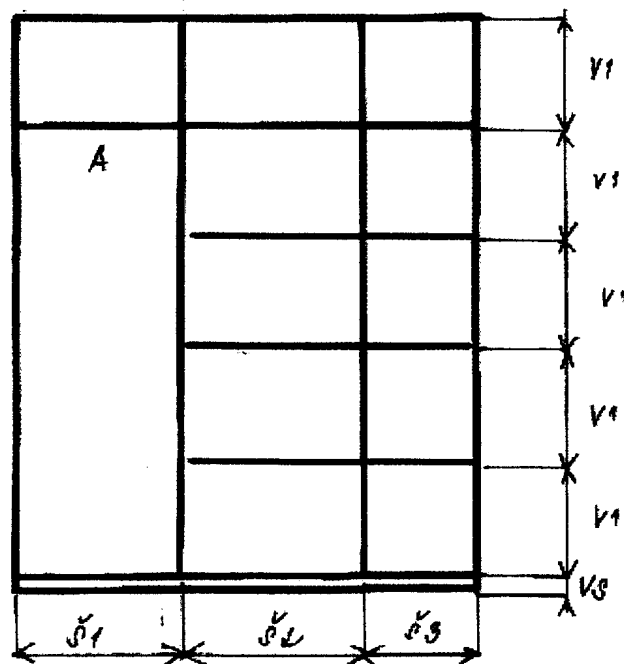
Vnitřní členění skříně
