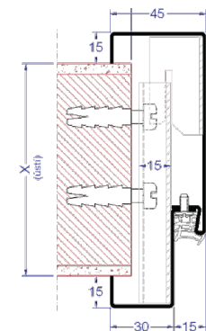
ILUSTRÁČNÍ SCHÉMA ZÁRUBNĚ
