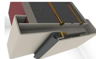
ILUSTRÁČNÍ FOTOGRAFIE ZÁRUBNĚ
