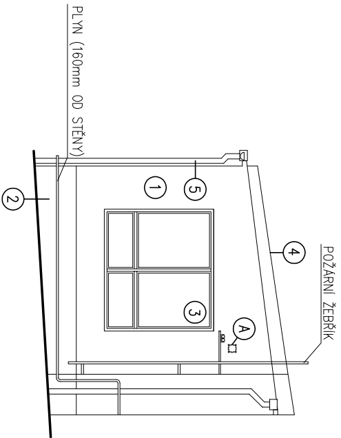
POHLED "B"
