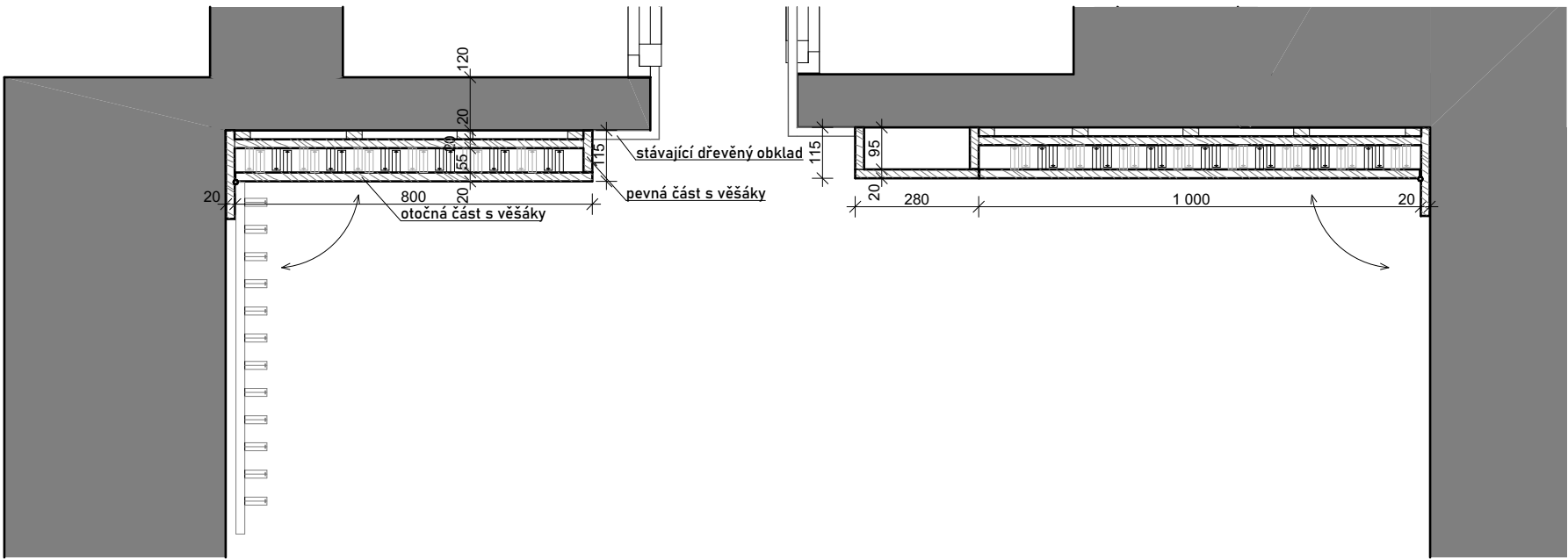
půdorys 1:15
