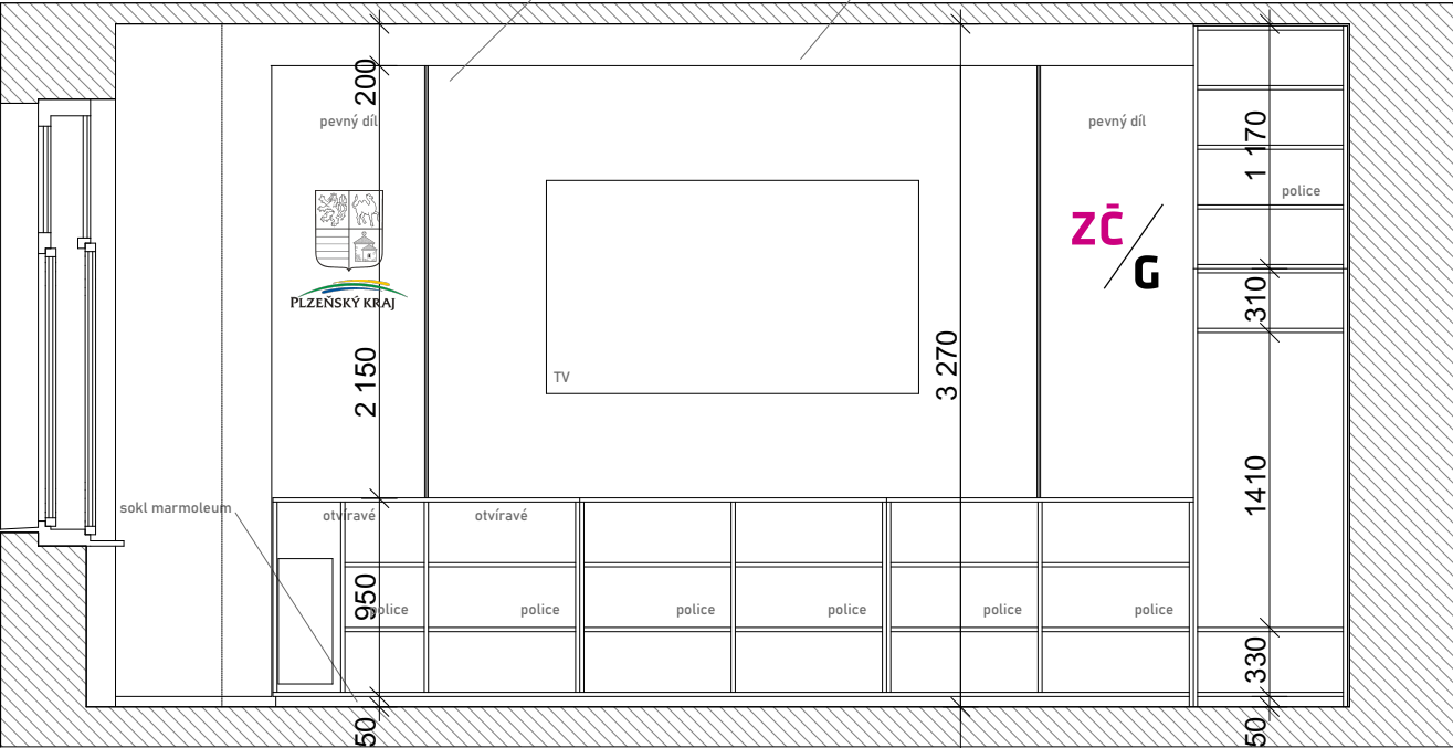
VNITŘNÍ USPOŘÁDÁNÍ
