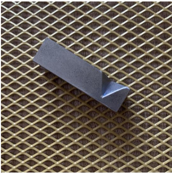
věšák tažený hranol - délka 55 mm, 14/14mm
